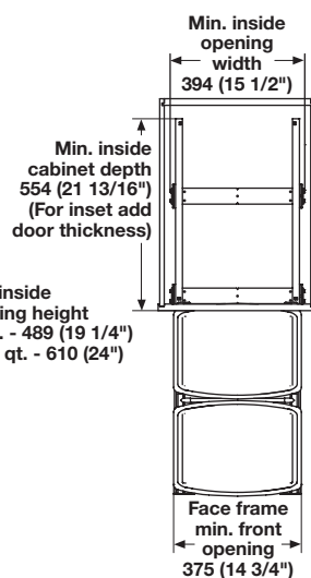
Double (2 x 36 qt.) (2 x 52 qt.)
